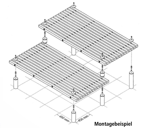
Montagebeispiel
